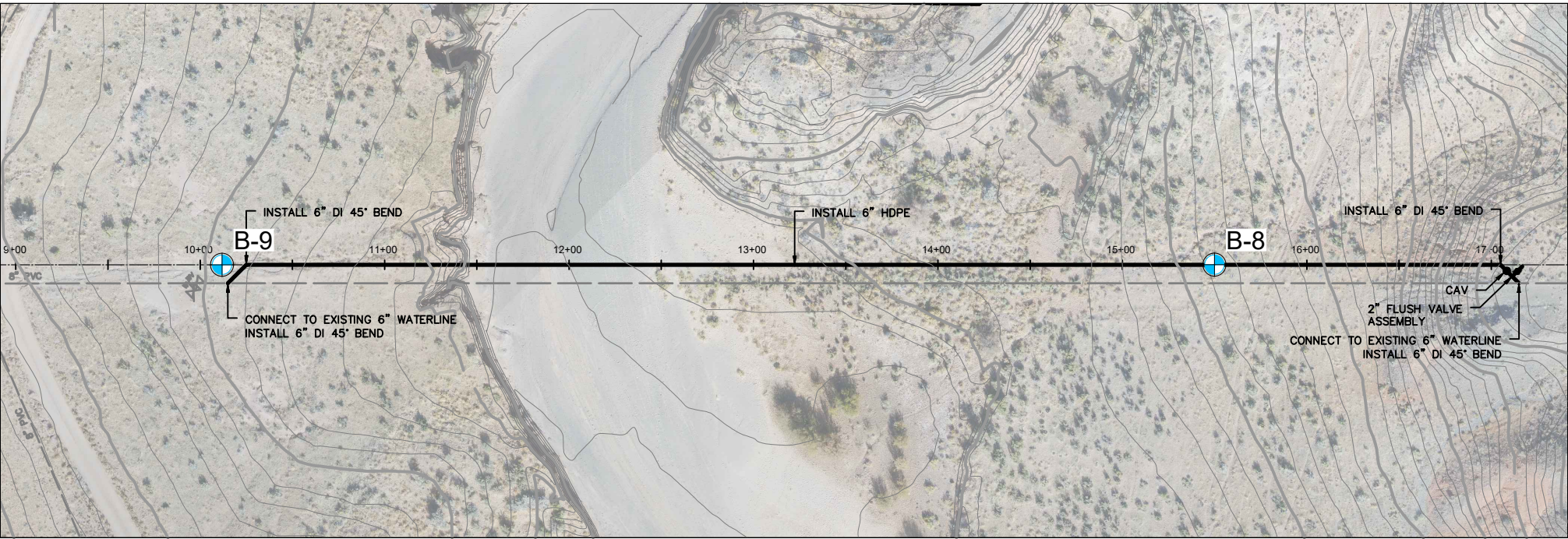
STA 10+00 - STA 17+00 PLAN
