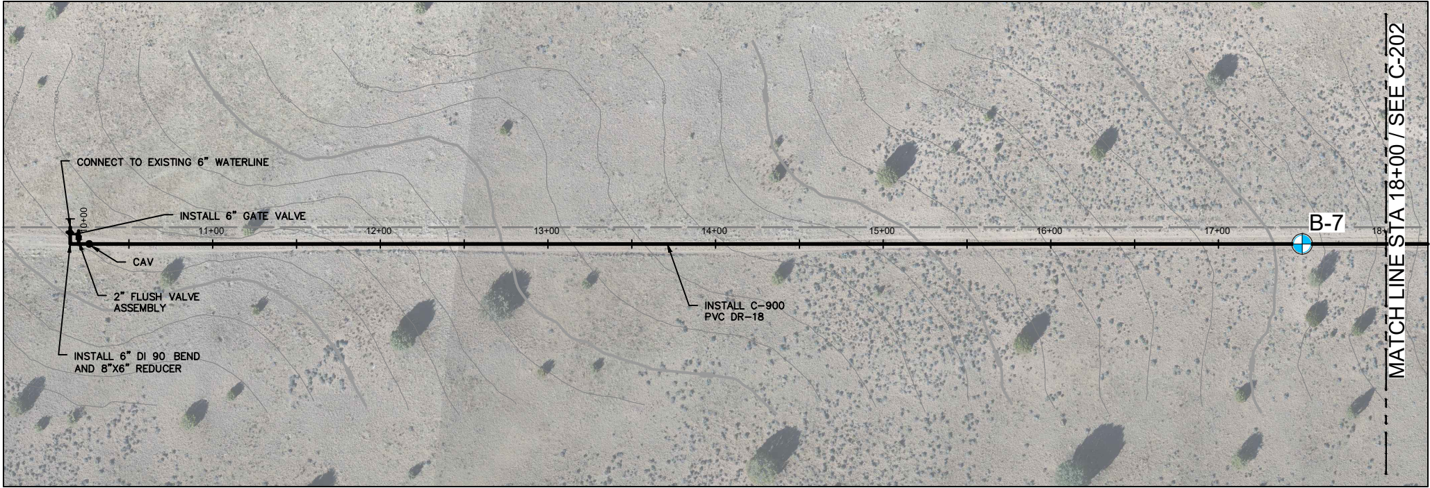
STA 10+00 - STA 18+00
