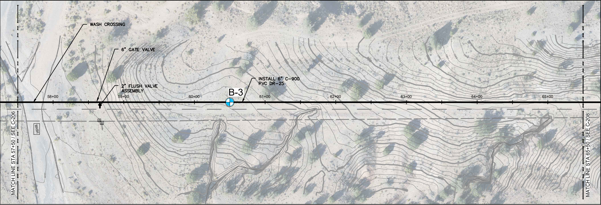
STA 57+50 - STA 65+50 PLAN
